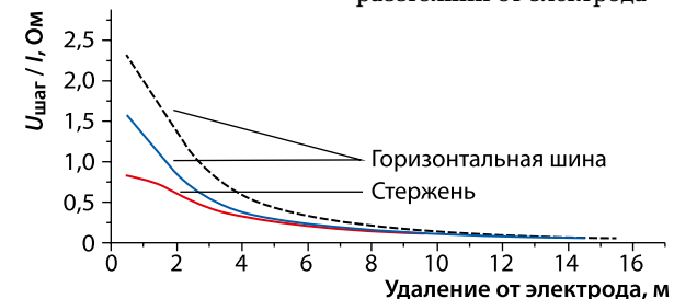
Рис. 2. Расчетные кривые Отношение напряжения шага ( U_{\text{шаг}} ) к току ( I ) на различном расстоянии от электрода
