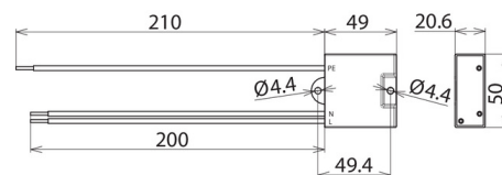
Размерный эскиз DCOR L 2P 275
