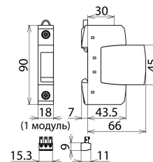
Размерный эскиз DGP C S FM
