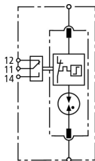
Принципиальная схема DGP C S FM
