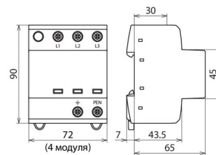
Размерный эскиз DSH TNC 255
