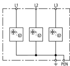
Принципиальная схема DSH TNC 255
