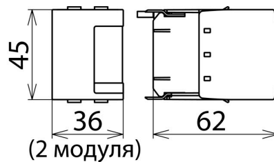
Размерный эскиз DV MOD 255
