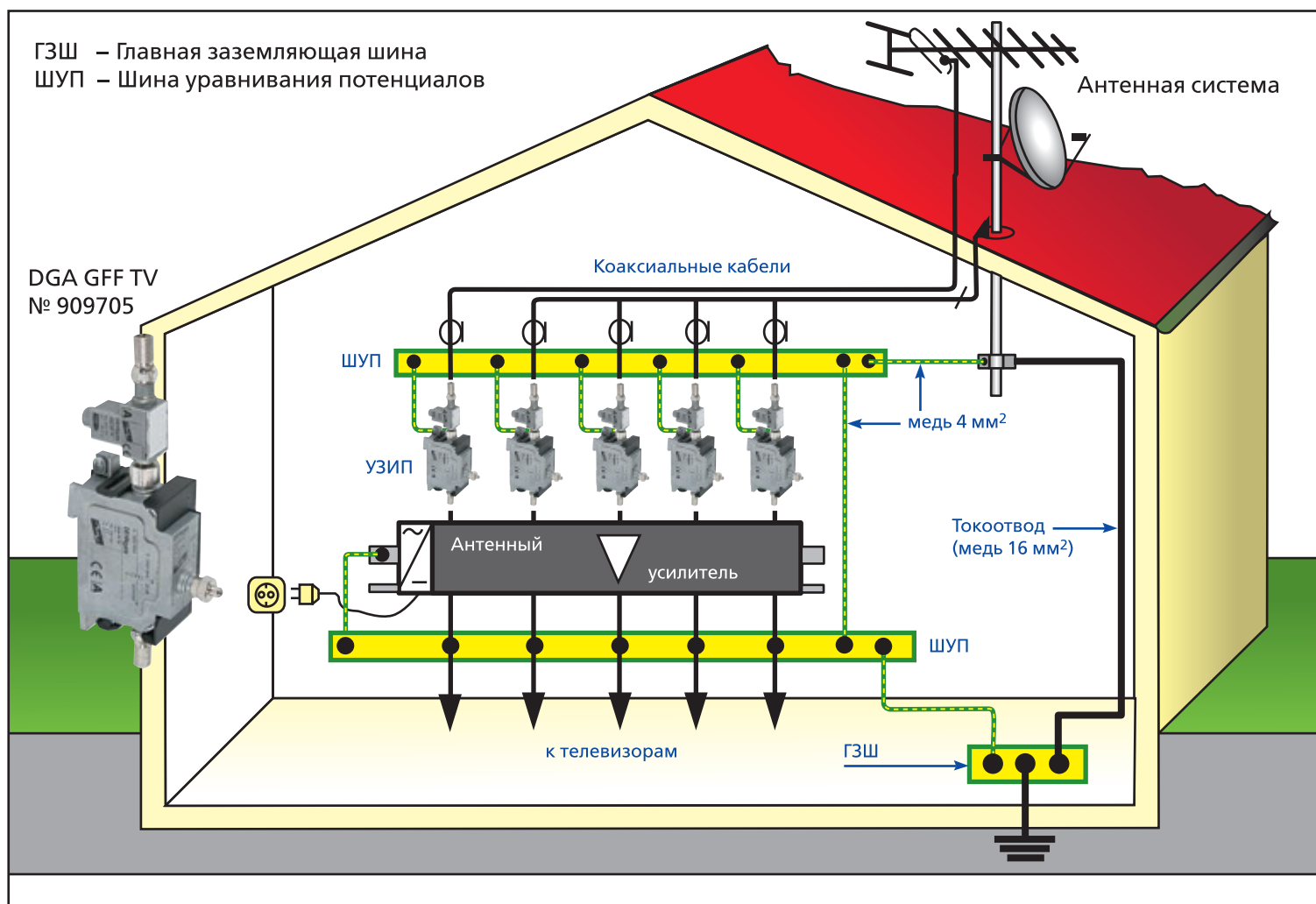
Рис. 1. Организация защиты антенны (на примере комплектующих производства фирмы Dehn+Söhne)
